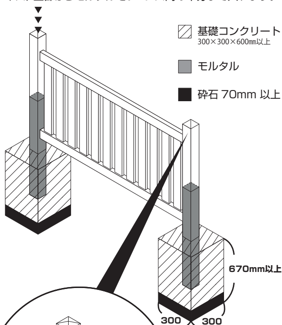
図④ ポスト上部からモルタルをフェンス高の半分まで入れます。
